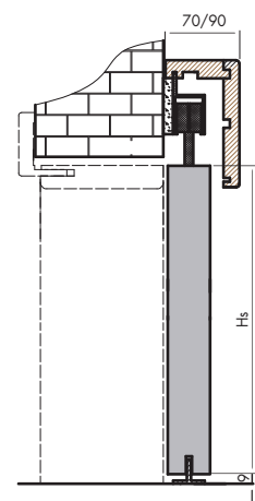
przekrój pionowy
