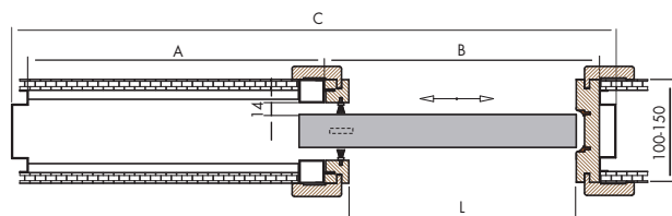
jednodzielne / przekrój poziomy
