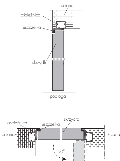
otwierane do wewnątrz 90^\circ
