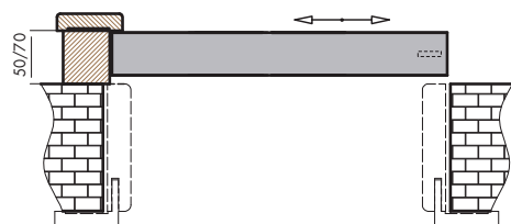
jednodzielne / przekrój poziomy
