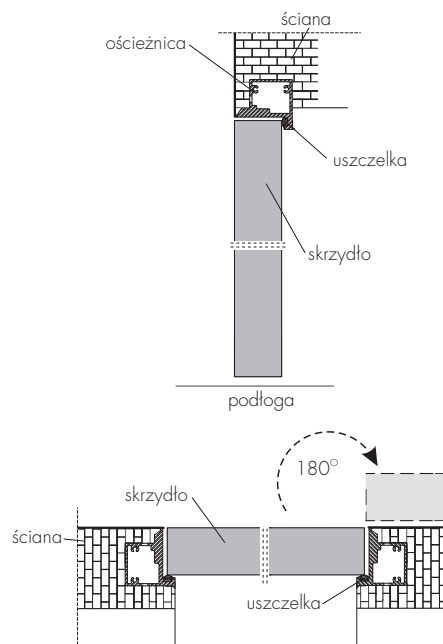
otwierane na zewnątrz 180^\circ
